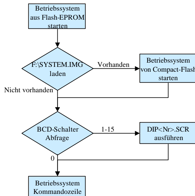
Abbildung 3: Boot-Vorgang
